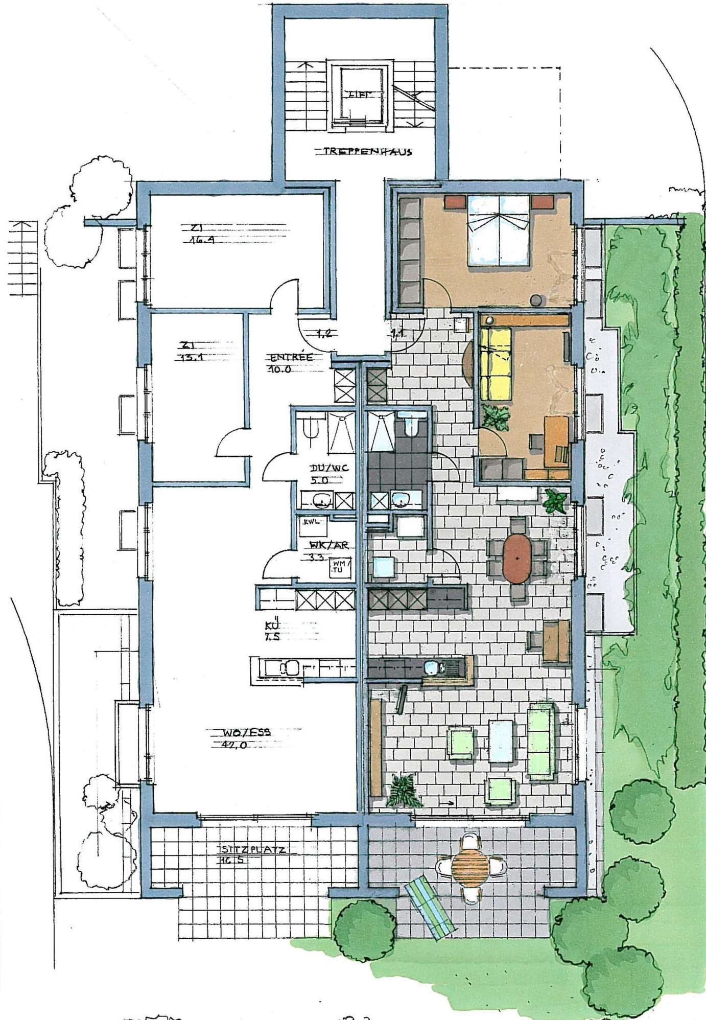
Grundriss Erdgeschoss
